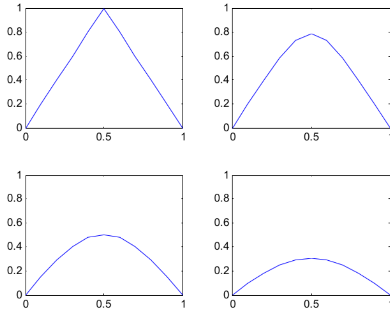
Gambar 4 Solusi numerik dari persamaan konduksi
