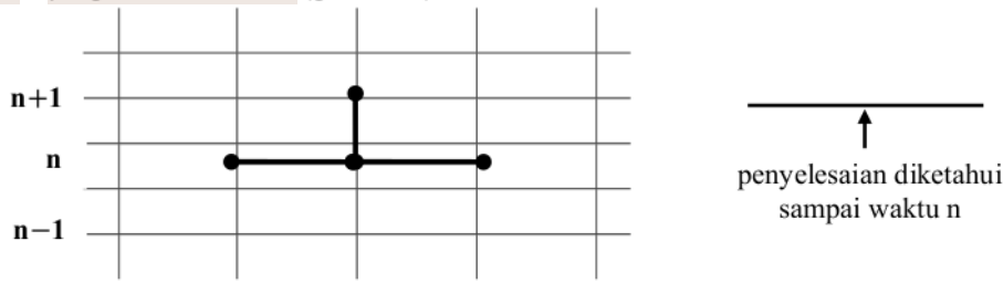
Gambar 3. Skema eksplisit
