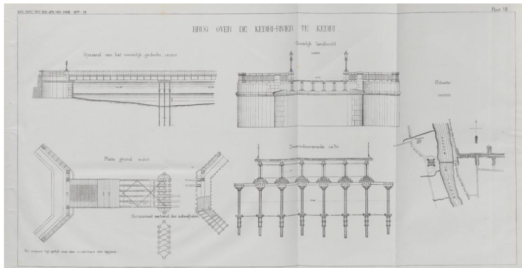
Gambar 1.9 Desain Jembatan Lama
