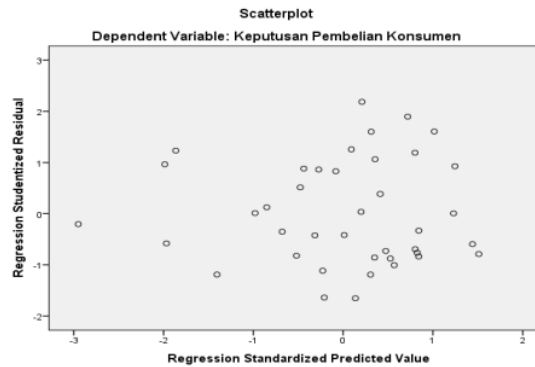
Gambar 2. Uji Heteroskedastisitas Sumber : data yang diolah, 2023
