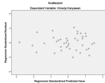
51 Grafik 2. Hasil Uji Heteroskedastisitas
