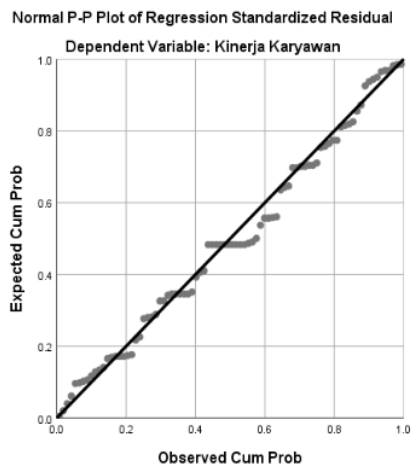
Gambar 1. Uji Normalitas
