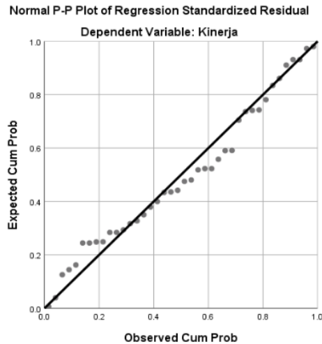
Gambar 1. Uji Normalitas Grafik P-P Plot
