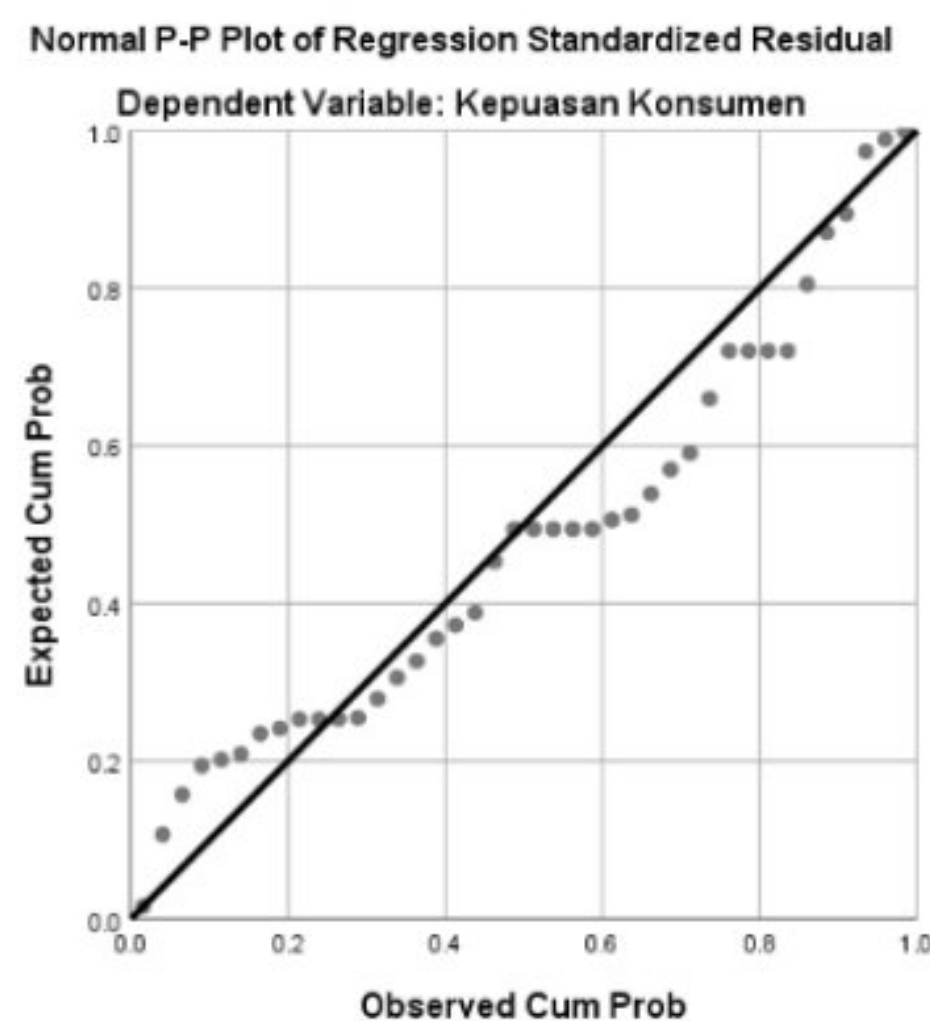
Gambar 1. Hasil Uji Normalitas
