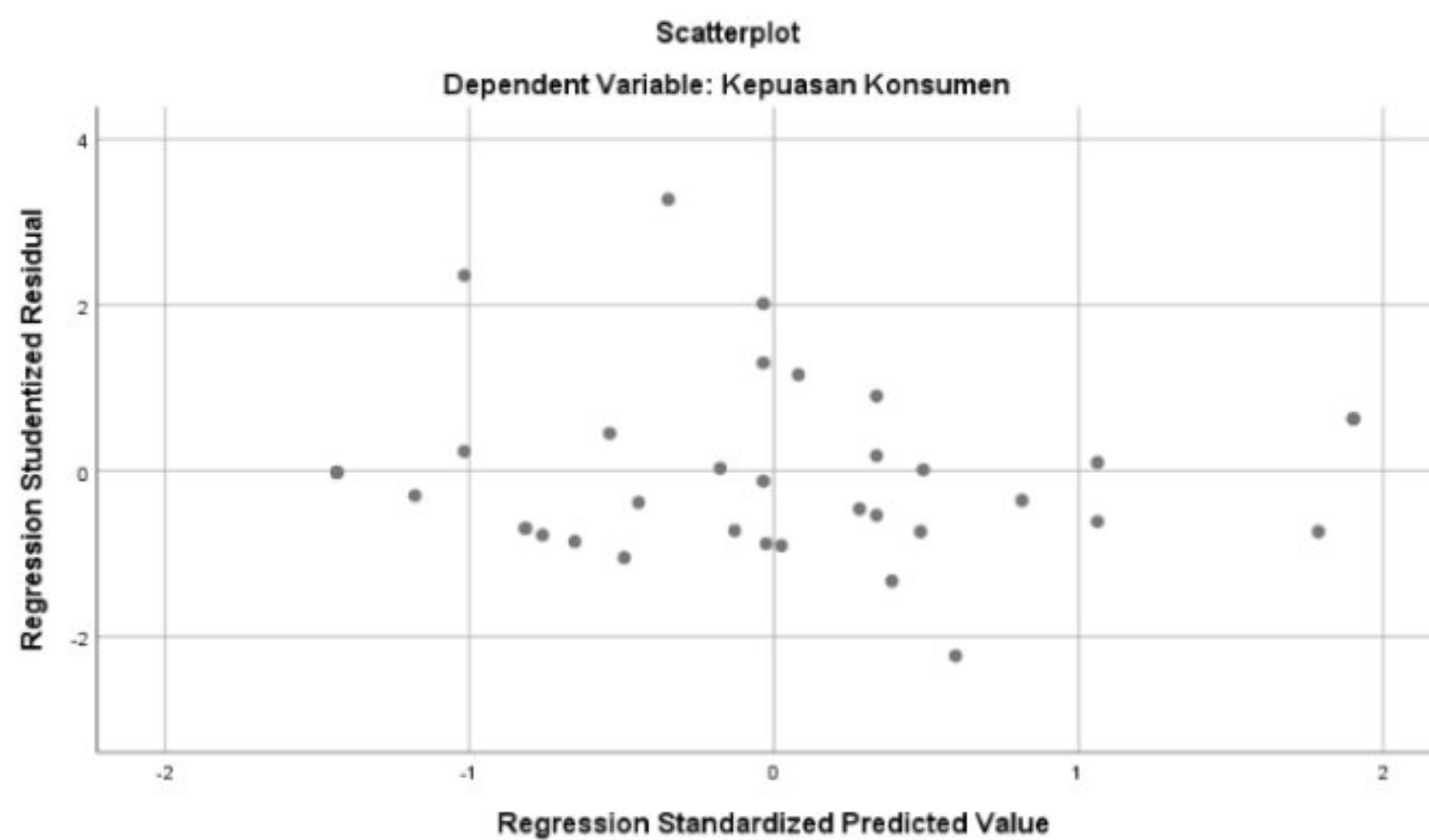
Gambar 2. Hasil Uji Heteroskedastisitas
