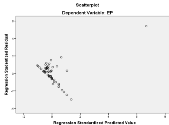
Gambar 2. Grafik Scatterplot
