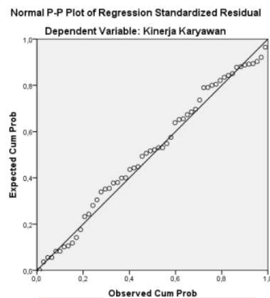
Gambar 1. Pengujian Normalitas
