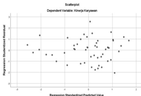
Gambar 2. Pengujian Heteroskedastisitas
