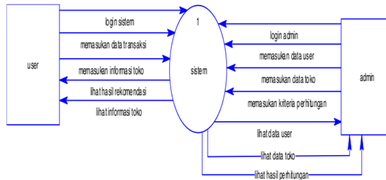
Gambar 2.2 Diagram Konteks
