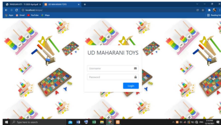
Gambar 4.1 Halaman Login
