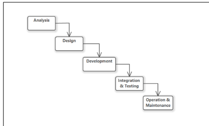
Gambar 1.1 Tahap Waterfall
