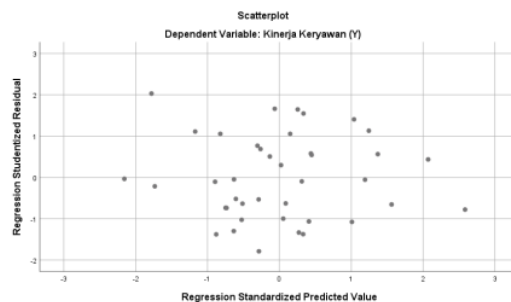
Gambar 2. Uji Heterokedastistas
