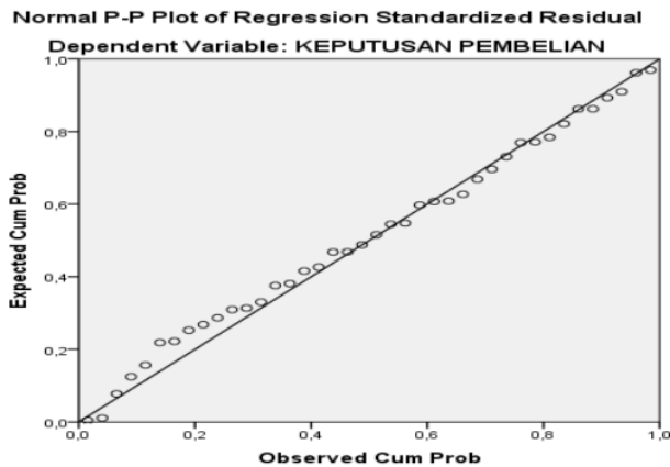
Gambar 1. Uji Normalitas 47
