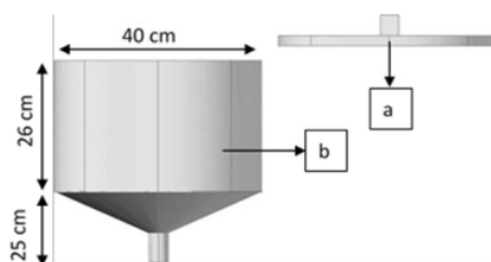
Gambar 3. Desain Wadah Penampung Pelet Ikan
