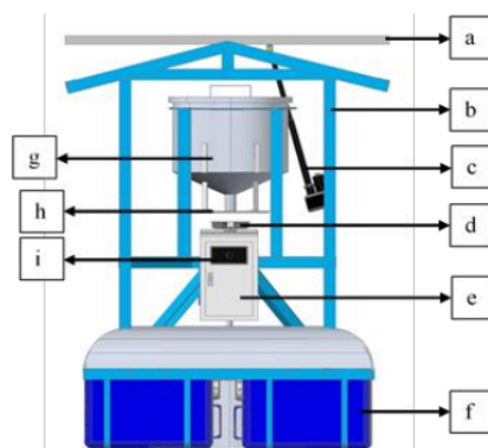
Gambar 2. Desain Alat Pelontar
