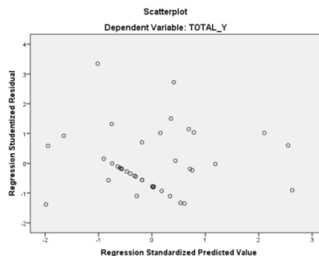
Gambar 2 Uji Heteroskedasitas
