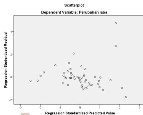
19 Gambar 2. Hasil Uji Heteroskedastisitas
