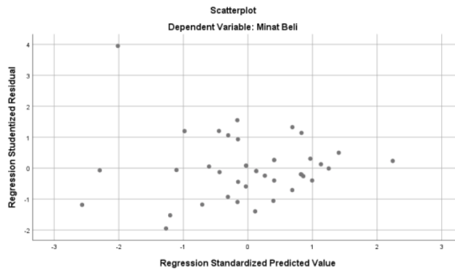
Gambar. 2 Grafik scatterplot
