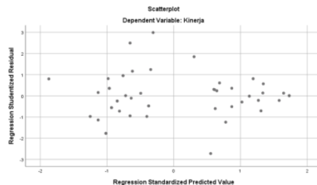
Gambar 4. Uji Heteroskedastisitas
