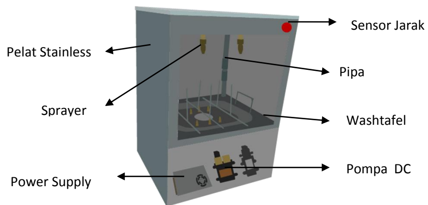
Gambar 1. Desain alat pencuci gelas otomatis berbasis arduino nano
