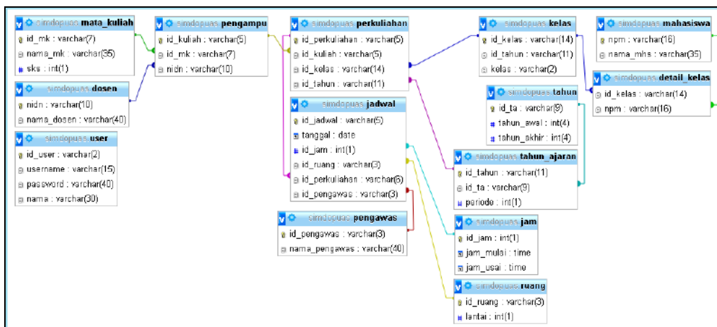
Gambar 2. Rancangan database
