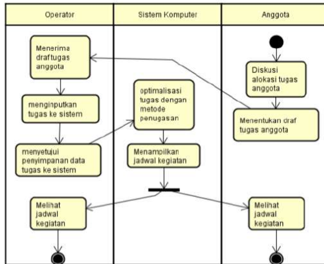
Gambar 4. Activity Diagram Membuat Alokasi Tugas
