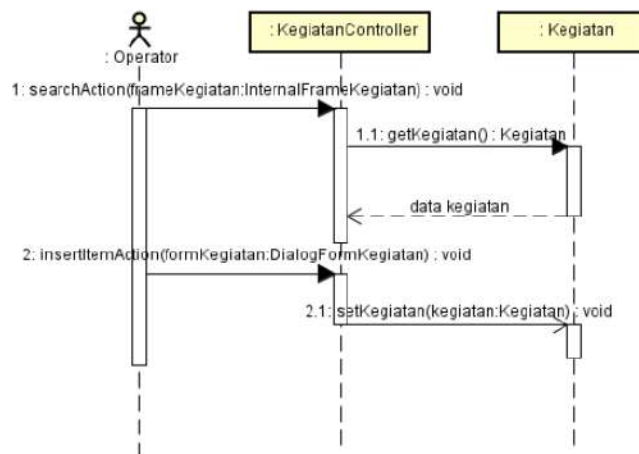
Gambar 6. Sequence Diagram Membuat Jadwal Kegiatan
