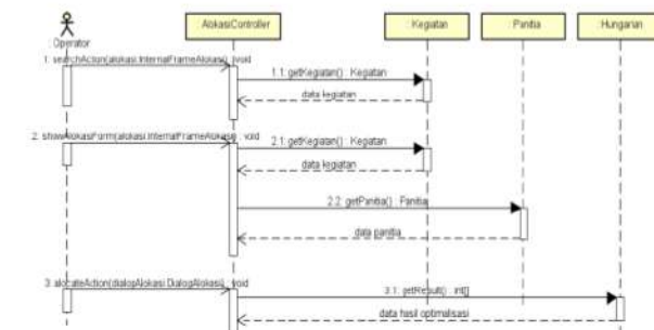
Gambar 7. Sequence Diagram Membuat Alokasi Tugas
