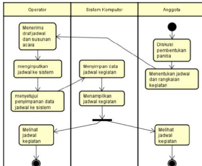
Gambar 3. Activity Diagram Membuat Jadwal Kegiatan
