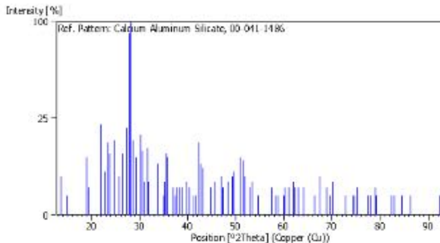
Gambar 4. Identifikasi fasa anorthite ( CaAl_2Si_2O_8 ) sampel pertama
