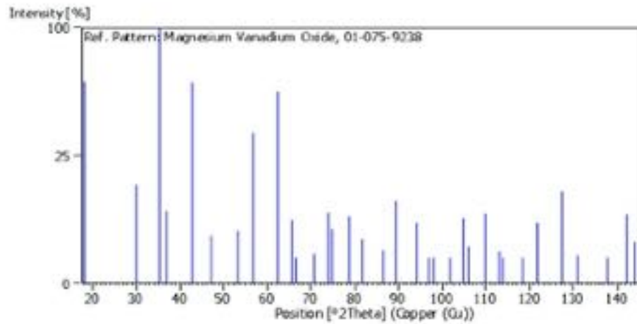
Gambar 7. Identifikasi fasa Magnesium Vanadium Oxide sampel kedua
