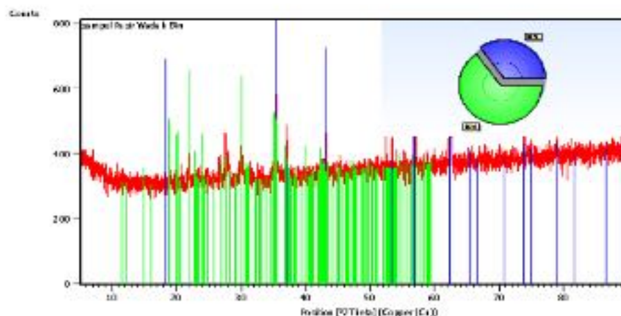
Gambar 6. Pola XRD sampel pasir besi sungai Drantas di lokasi kedua
