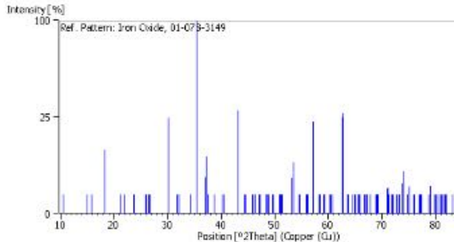
Gambar 5. Identifikasi fasa magnetit ( \text{Fe}_3\text{O}_4 ) sampel pertama
