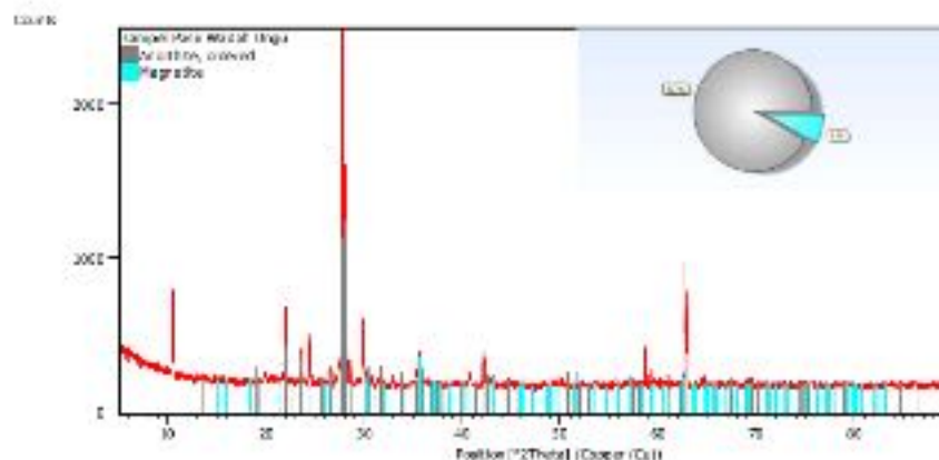
Gambar 2.2 Pola XRD sampel pasir besi sungai Brantas
