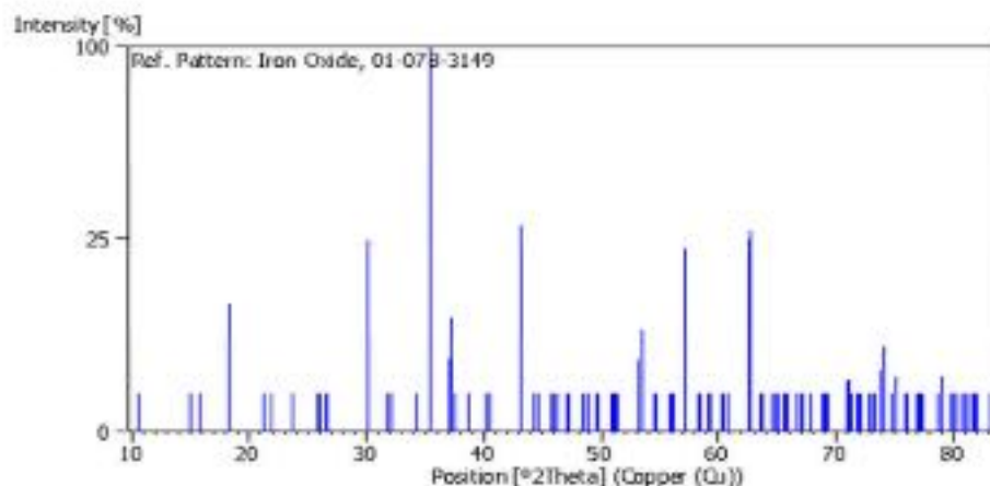
Gambar 2.4 Identifikasi fasa magnetit ( \text{Fe}_3\text{O}_4 )
