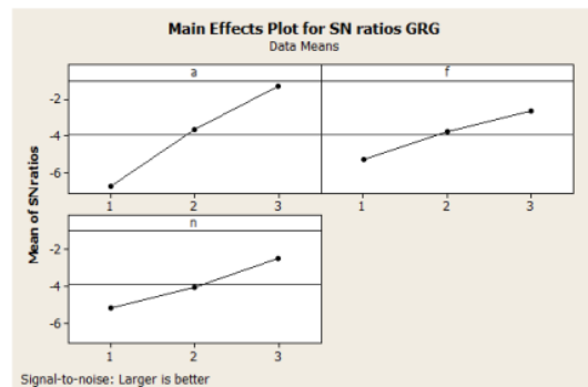
Gambar 4. Main effect plot untuk S/N Ratio GRG
