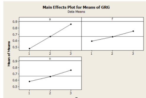
Gambar 3. Main effect plot untuk rata-rata GRG
