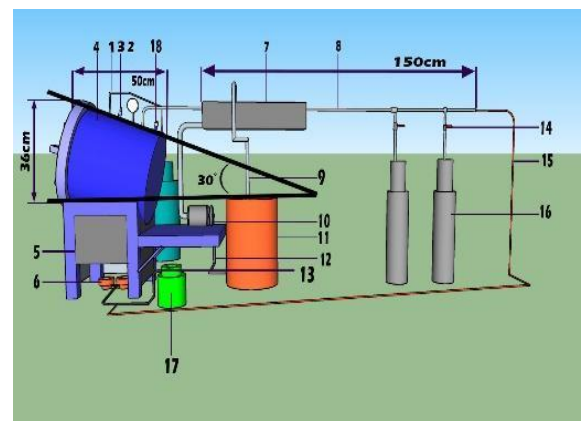
Gambar 4. Alat pirolisis
