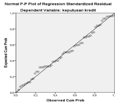
Gambar 1 25 Uji Normalitas
