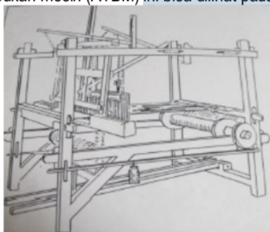
Gambar 1. Alat Tenun Bukan Mesin (ATBM) (Herlison Enie, 1980: 7)
