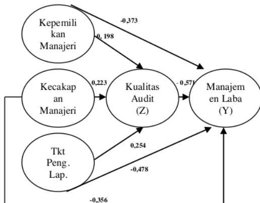
Gambar.1. Diagram hasil analisis jalur
