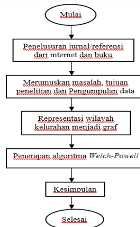
Gambar 1. Tahapan penelitian
