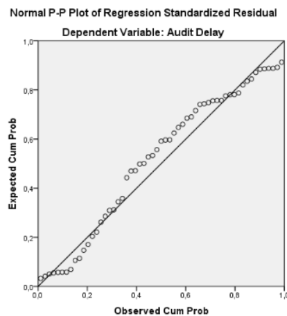
Gambar 2 Normal P-Plot Setelah Outlier
