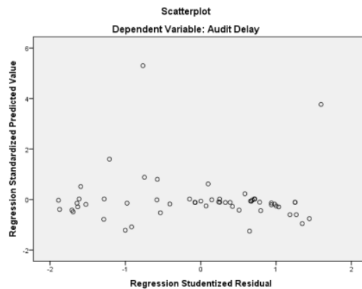
Gambar 3 Grafik Scatterplot
