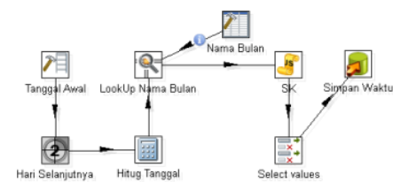
Gambar 8. Transformasi Ke D imensi Waktu
