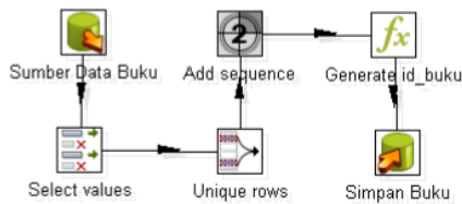
Gambar 5. Transformasi Ke Dimensi Buku
