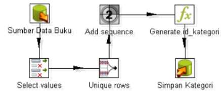
Gambar 7. Transformasi Ke Dimensi Kategori
