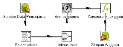
Gambar 6. Transformasi Ke Dimensi Anggota
