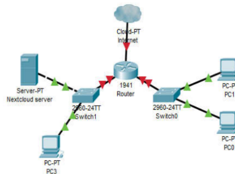
Gambar.3 topologi usulan
