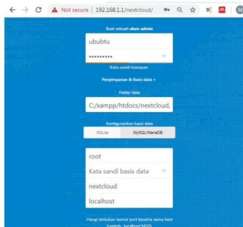
Gambar 6. Konfigurasi Nextcloud
