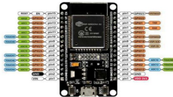
Gambar 2. 2 Spesifikasi Esp32
