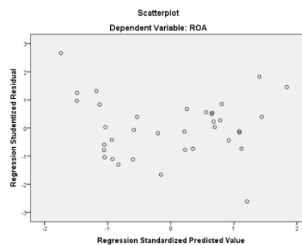
Gambar 1. Hasil Uji Heterokedastisitas Grafik Scatterplots
