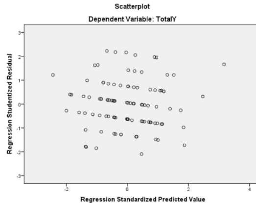
Sumber : data primer diolah, 2023 Gambar 2. Hasil Uji Heteroskedastisitas
