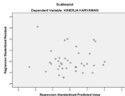
Gambar 2 Grafik Scaterplots
