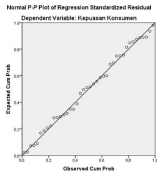
Gambar 1 Hasil Uji Normalitas Sumber : data yang diolah, 2023
