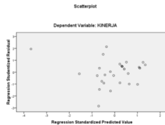
Gambar 8. Hasil Uji Heteroskedastisitas Grafik Scatterplots
