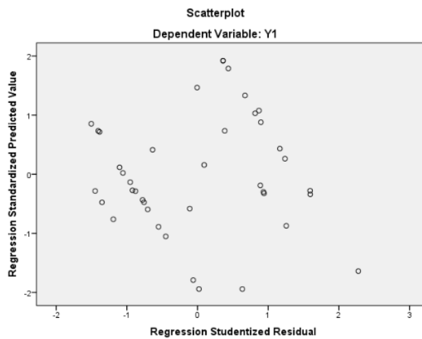
Gambar 1 Uji Heteroskedastisitas Sumber : Data primer diolah SPSS v.23 2023
