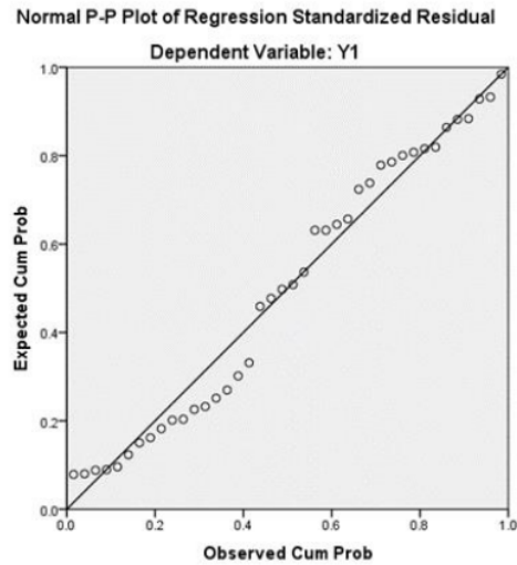
61 Gambar 1 Uji Normalitas Sumber : Output SPSS v.23
