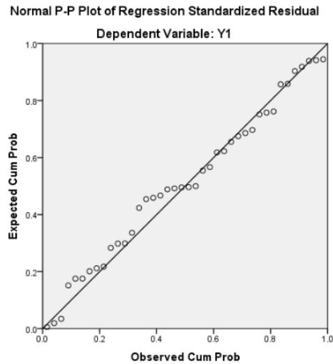
Gambar 1 Uji Normalitas Sumber : Output SPSS v.23
