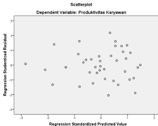
Sumber : Data primer yang diolah, 2023 Gambar 2. Hasil Uji Heteroskedastitas
