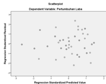
Gambar 2 Hasil Uji Heterosiditas
