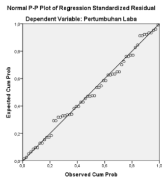
Sumber : Output SPSS Versi 23 Gambar 1 Hasil Uji Normalitas
